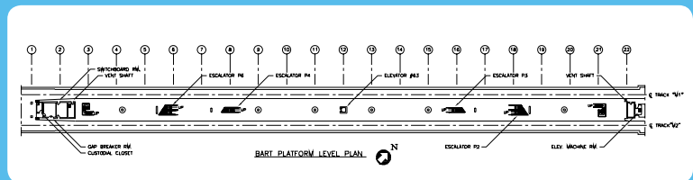
Embarcadero 站 - 平台平面方案
