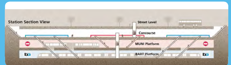
Embarcadero 站 - 側視圖
