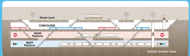
Montgomery 站 - 側視圖
